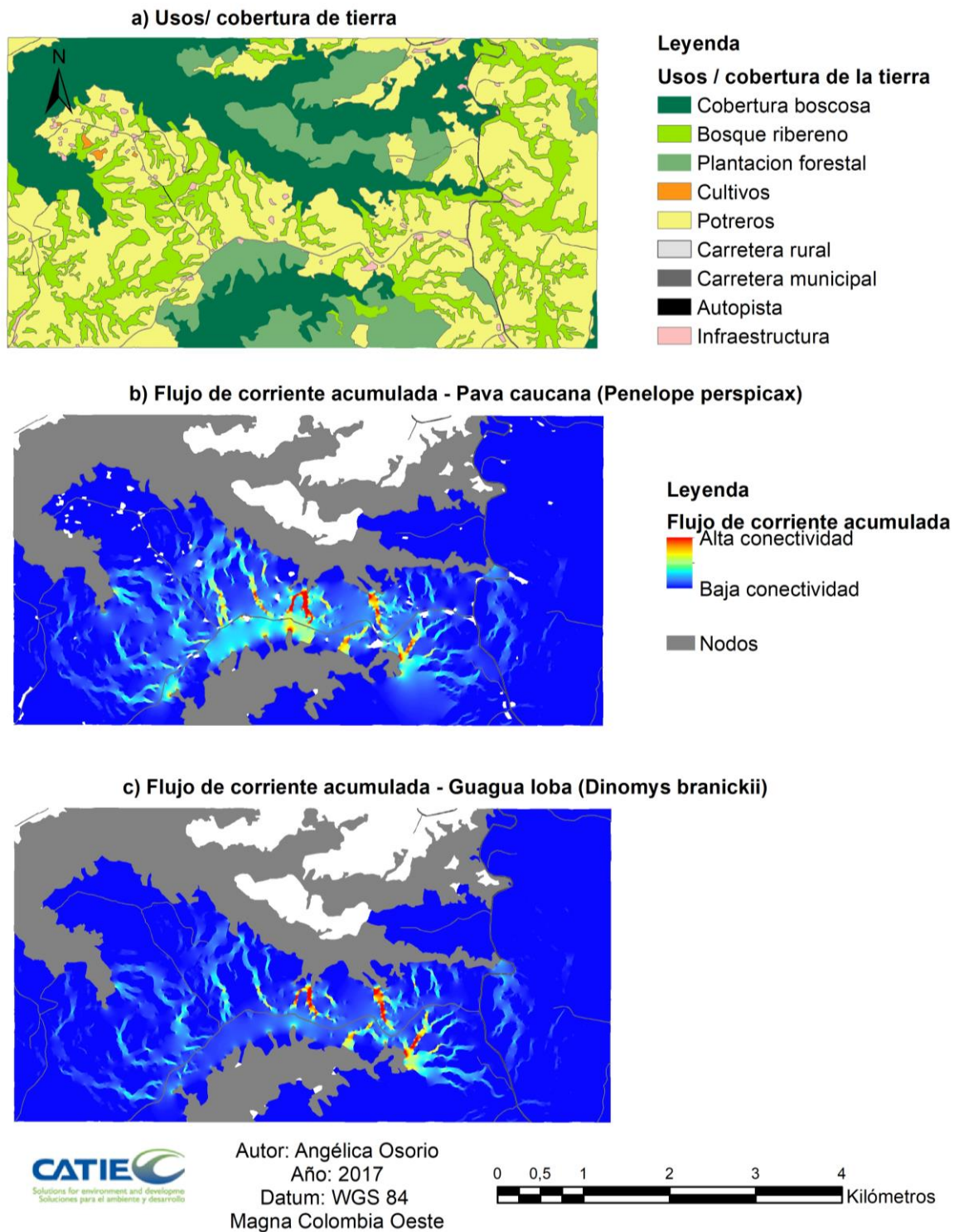
Figura 3. Año 2003 – Línea base: a) Mapa de usos/cobertura de la tierra, b) Modelo de flujo de corriente acumulada para la “pava caucana” ( Penelope perspicax ) y c) Modelo de flujo de corriente acumulada para la “guagua loba” ( Dinomys branickii ), cuenca media del cañón del río Barbas, Filandia y Pereira, Colombia Elaborado por Angélica Osorio, 2017.
