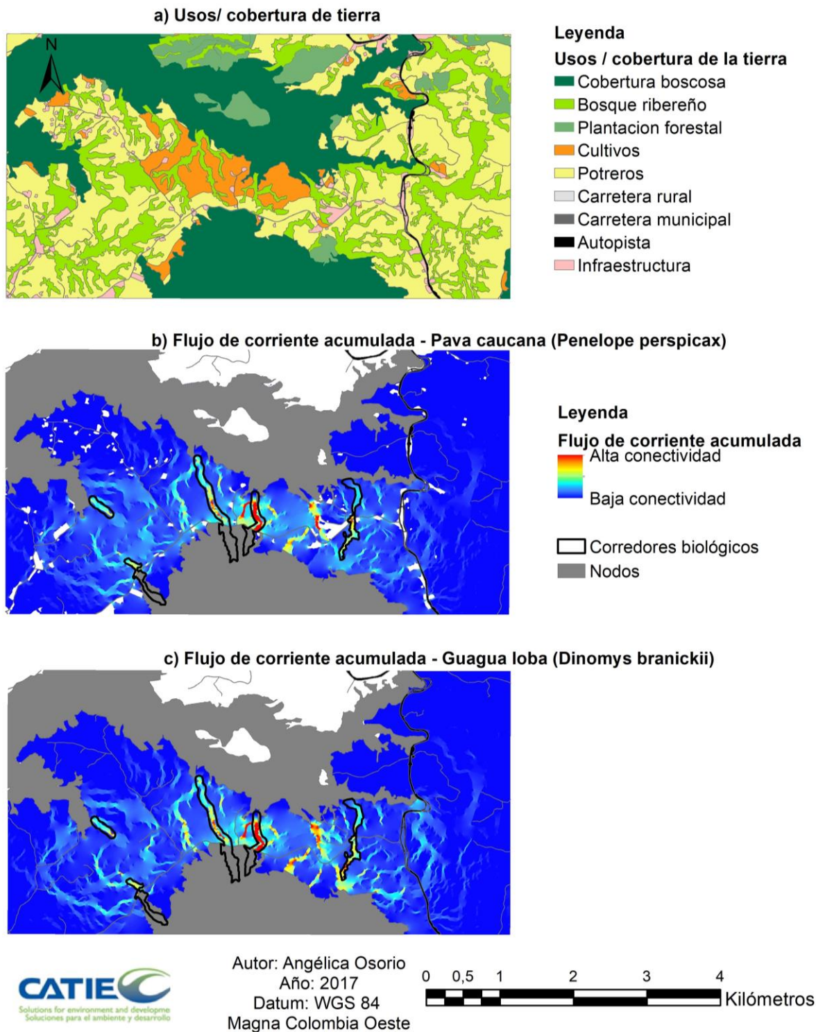
Figura 4. Año 2014: a) Mapa de usos/cobertura de la tierra, b) Modelo de flujo de corriente acumulada para la “pava caucana” ( Penelope perspicax ) y c) Modelo de flujo de corriente acumulada para la “guagua loba” ( Dinomys branickii ), cuenca media del cañón del río Barbas, Filandia y Pereira, Colombia .Elaborado por Angélica Osorio, 2017.
