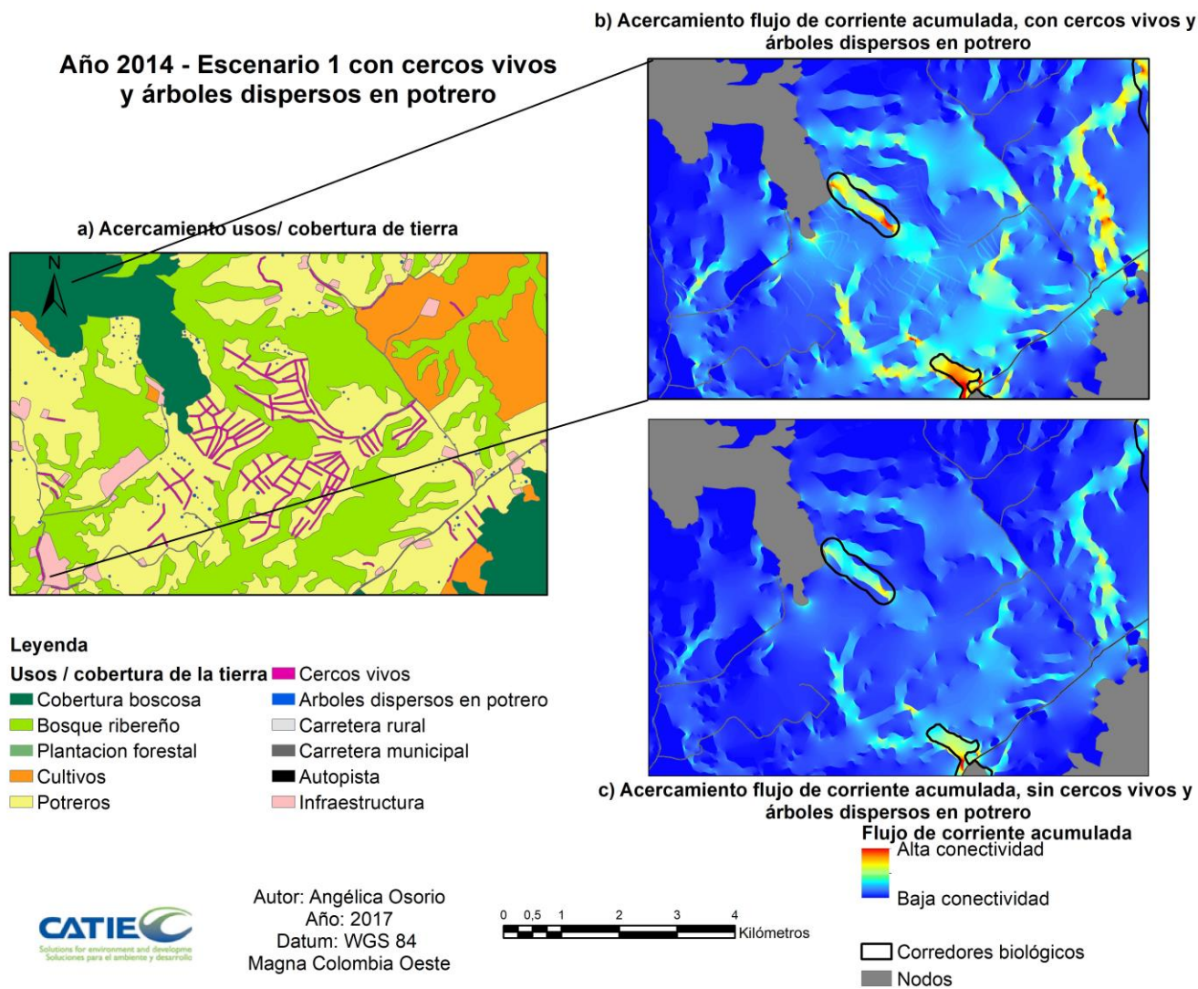
Figura 5. Año 2014 – Escenario 1 con cercos vivos y árboles dispersos en potrero: a) Mapa de usos/cobertura de la tierra, b) Acercamiento mapa de usos/cobertura de la tierra y c) Acercamiento modelo de flujo de corriente acumulada “pava caucana” ( Penelope perspicax ), cuenca media del cañón del río Barbas, Filandia y Pereira, Colombia. Elaborado por Angélica Osorio, 2017.
