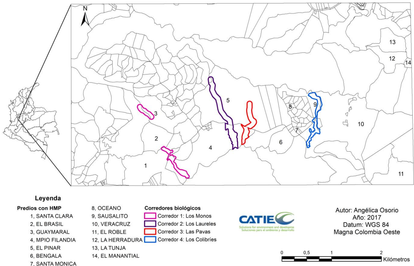
Figura 1. Ubicación del área de estudio, predios con HMP y corredores biológicos implementados en el municipio de Filandia, departamento del Quindío y Pereira, departamento de Risaralda, Colombia.
